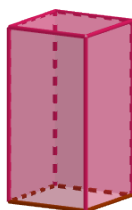
Prisma cuadrangular (irregular)
