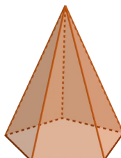
Pirámide pentagonal (irregular)
