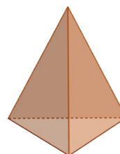
Pirámide triangular (irregular)
