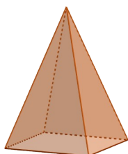
Pirámide cuadrangular (irregular)
