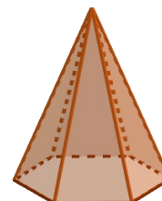
Pirámide hexagonal (irregular)
